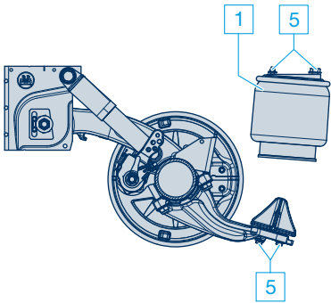
Versione con molla aria separata (Kombi airbag)
