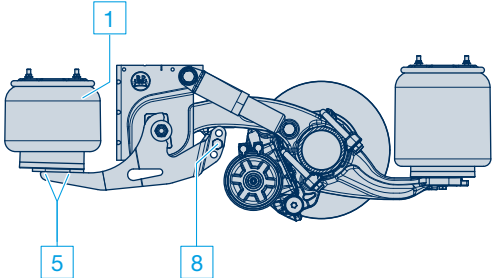
Sollevatore laterale
