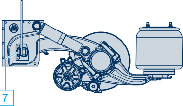
Rinforzi imbullonati al perno balestra
